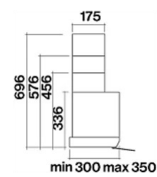
Optional chimney
